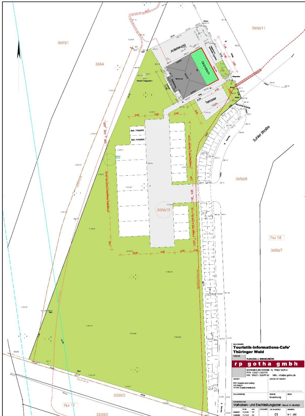
Abb. 10: Planzeichnung des Vorhaben- und Erschließungsplanes
